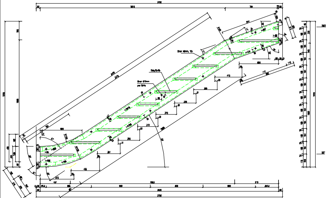
Schodnica S202/1 1:100
