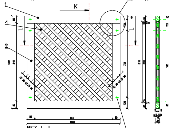
REZ L-L M 110
